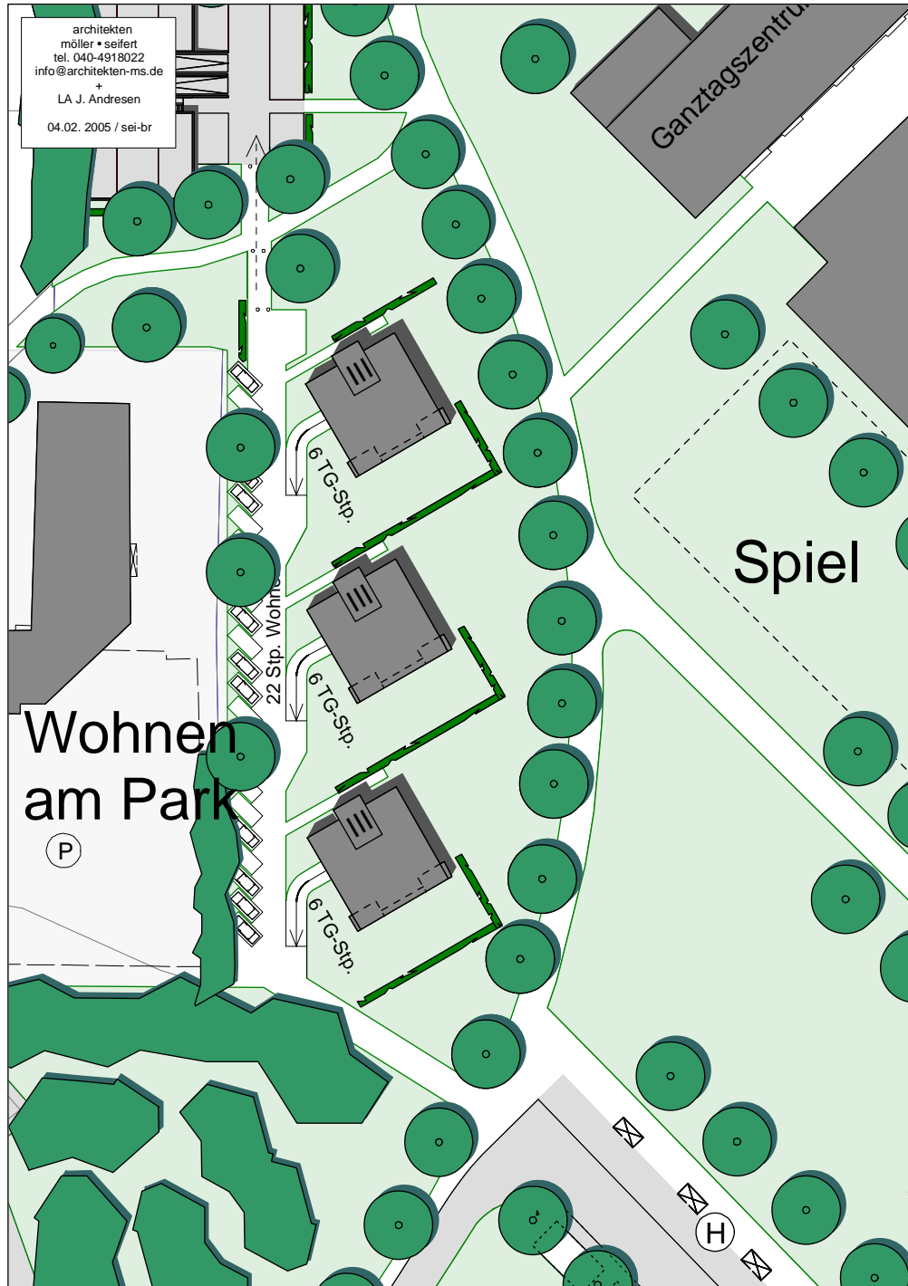
Lageplan Neubebauung Wohnen am Park Maßstab 1:500 (DIN A3)
